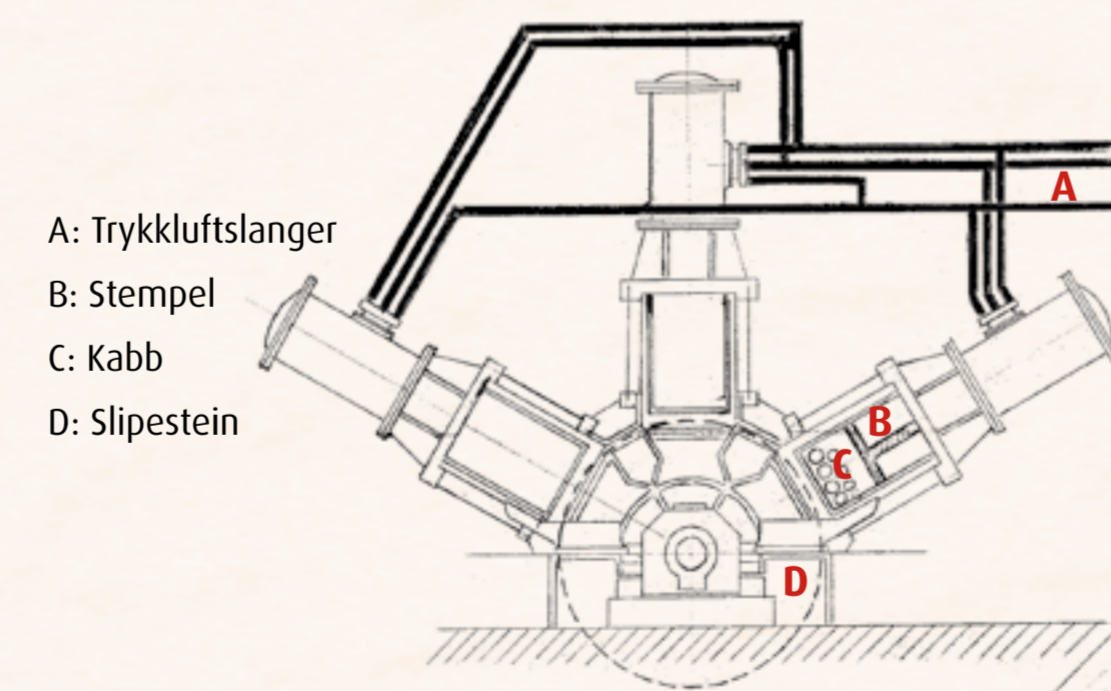
Teknisk tegning av Myrens ileggsapparat for varmslip, med tre ilegg. Utlånt av Trygve Hagen.
